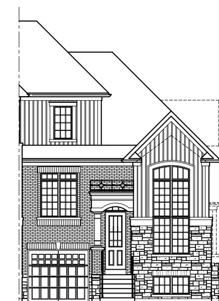
ELEVATION A
